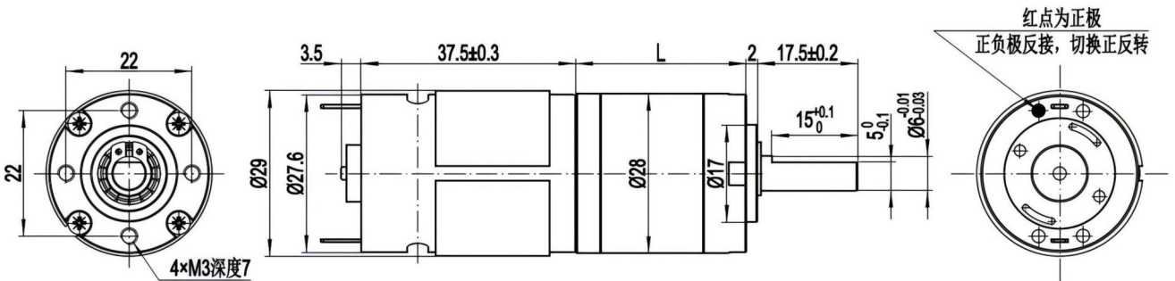
马达尺寸图 (单位: mm)
