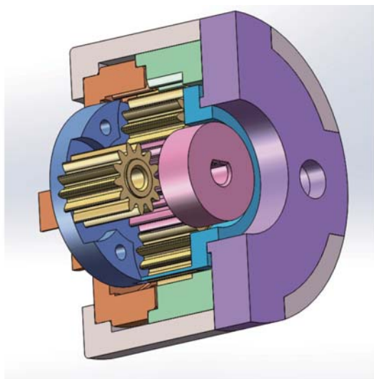
项目名称: NGWN型行星轮系
