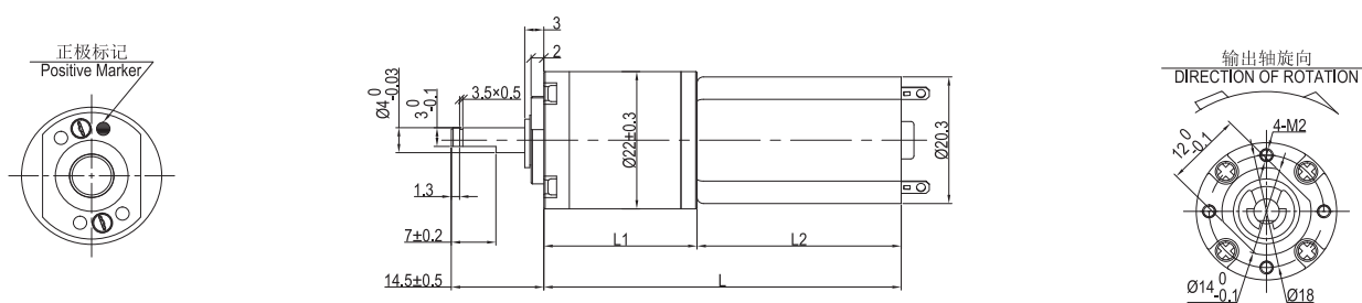
外形图 (单位 mm) Dimensions(Unit mm)
