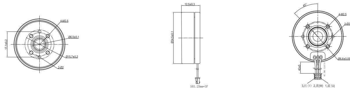
外形图 (单位 mm) Dimensions(Unit mm)
