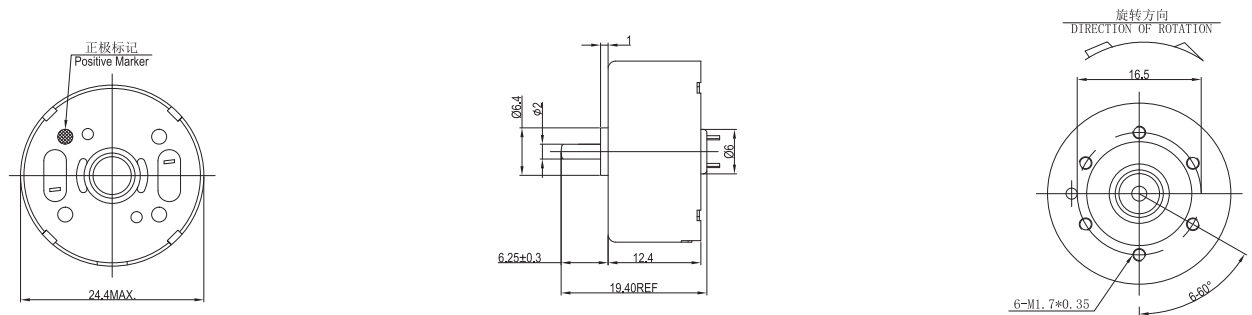
外形图（单位 mm） Dimensions(Unit mm)
